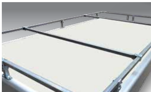
Barres transversales pour rails de transport vélos (2 pièces non montées)
