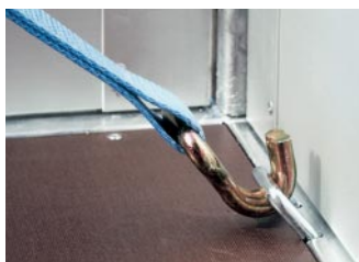
Anneau de fixation encastré
